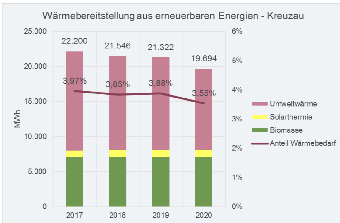
Abbildung 20: Wärmebereitstellung aus erneuerbaren Energien - Kreuzau
