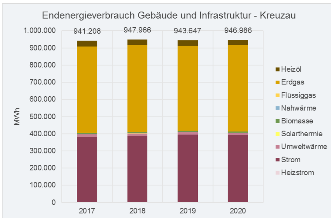
Abbildung 10: Endenergieverbrauch Gebäude und Infrastruktur - Kreuzau
